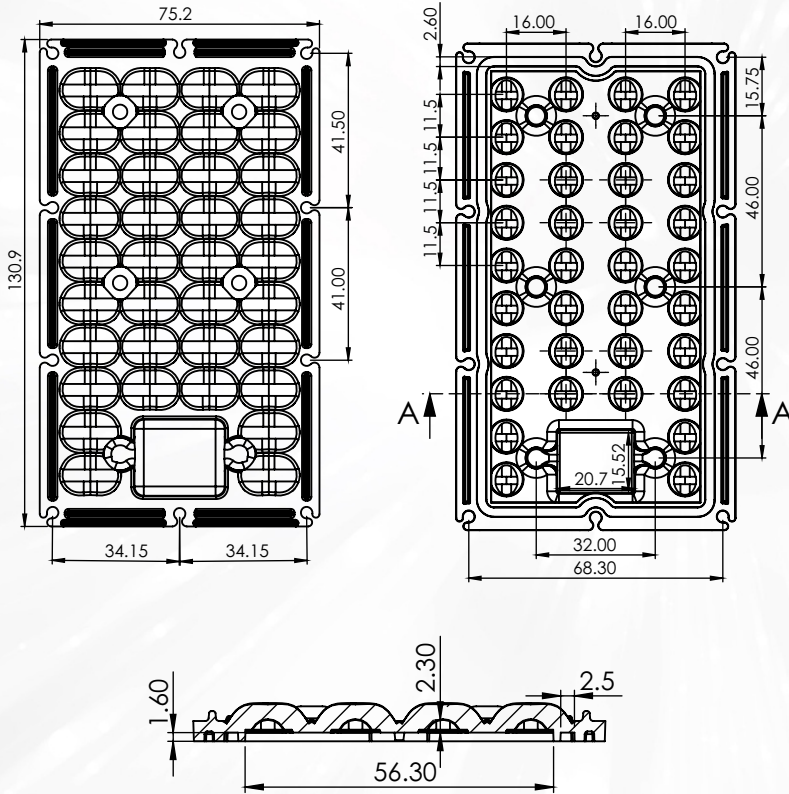
SECTION A-A
